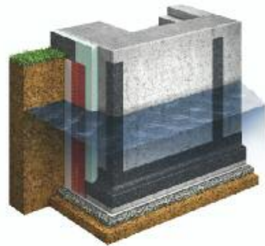
Laut dem VPB, dem Verband Privater Bauherren e. V., steigt mancherorts der Grundwasserspiegel an, ein Keller aus WU-Beton, die „Weiße Wanne“, sei ratsam. Hier mit zusätzlicher Abdichtung gegen drückendes Wasser. Glatthaar
